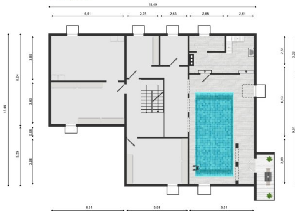
Grundriss Kellergeschoss (Grundriss)
